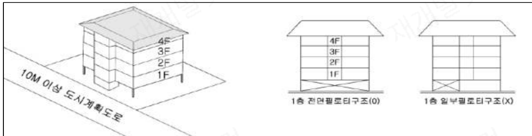
【그림1】 건축물 높이 예시도(제1종일반주거지역, 10m이상 도시계획도로와 접한 경우)
