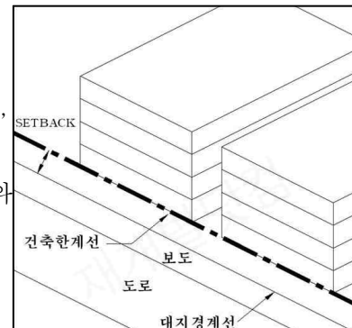
【그림2】 건축한계선
