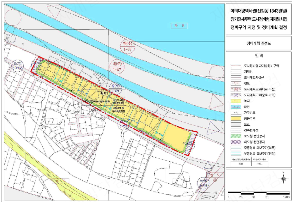
< 정비계획 결정도 >
