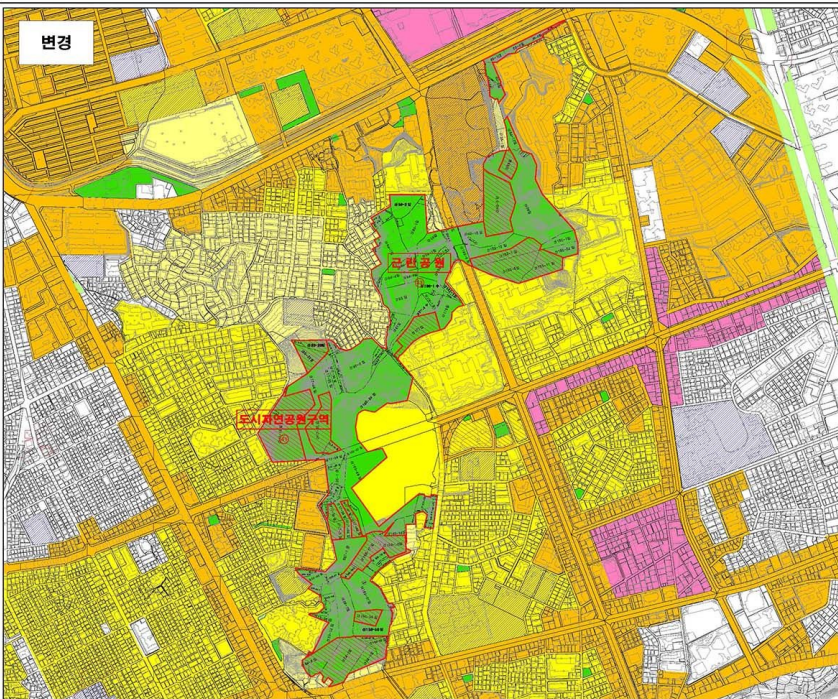
■ 도시관리계획 결정도
