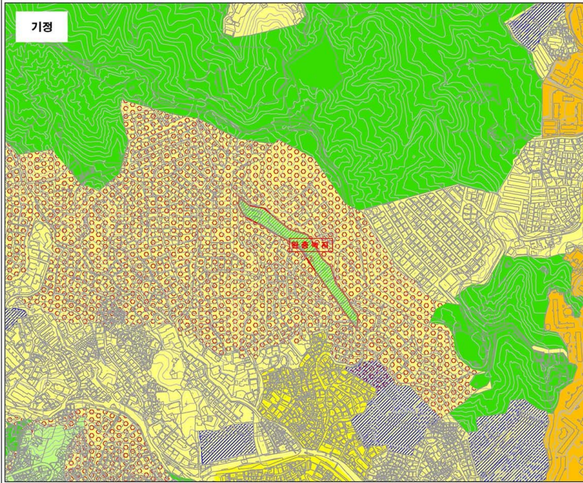
■도시관리계획 결정도
