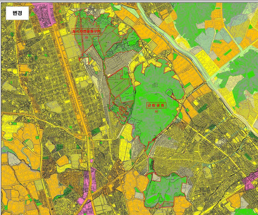
■ 도시관리계획 결정도
