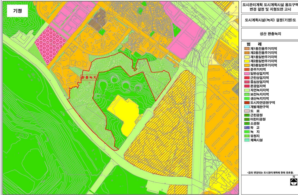
■도시관리계획 결정도
