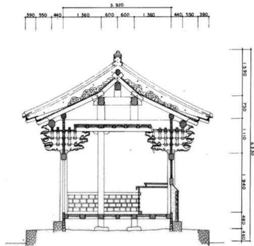
그림 12. 칠성각 단면도 (서울특별시, 1990)
