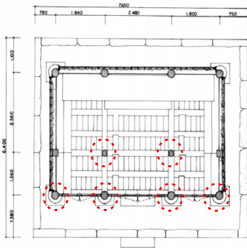
그림 11. 칠성각 평면도 (서울특별시, 1990)
