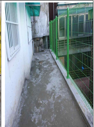
공사시행완료 - 옹벽상단 배수구 설치, 바닥 방수
