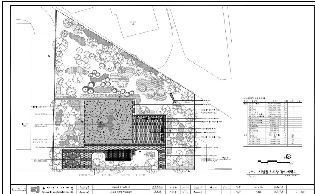
공사설계도서(시설물/포장정비 계획도)
